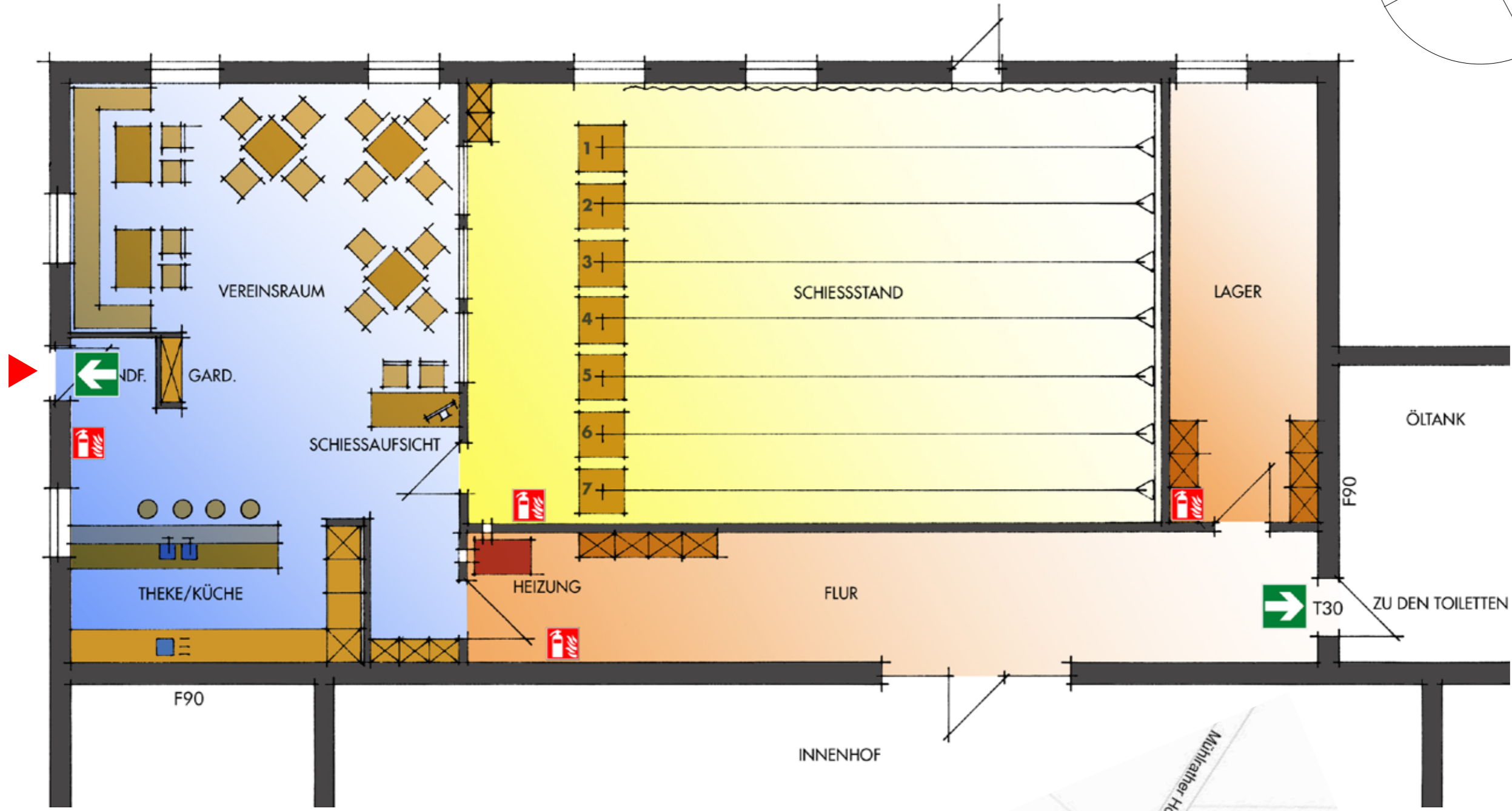
GRUNDRISS ERDGESCHOSS
